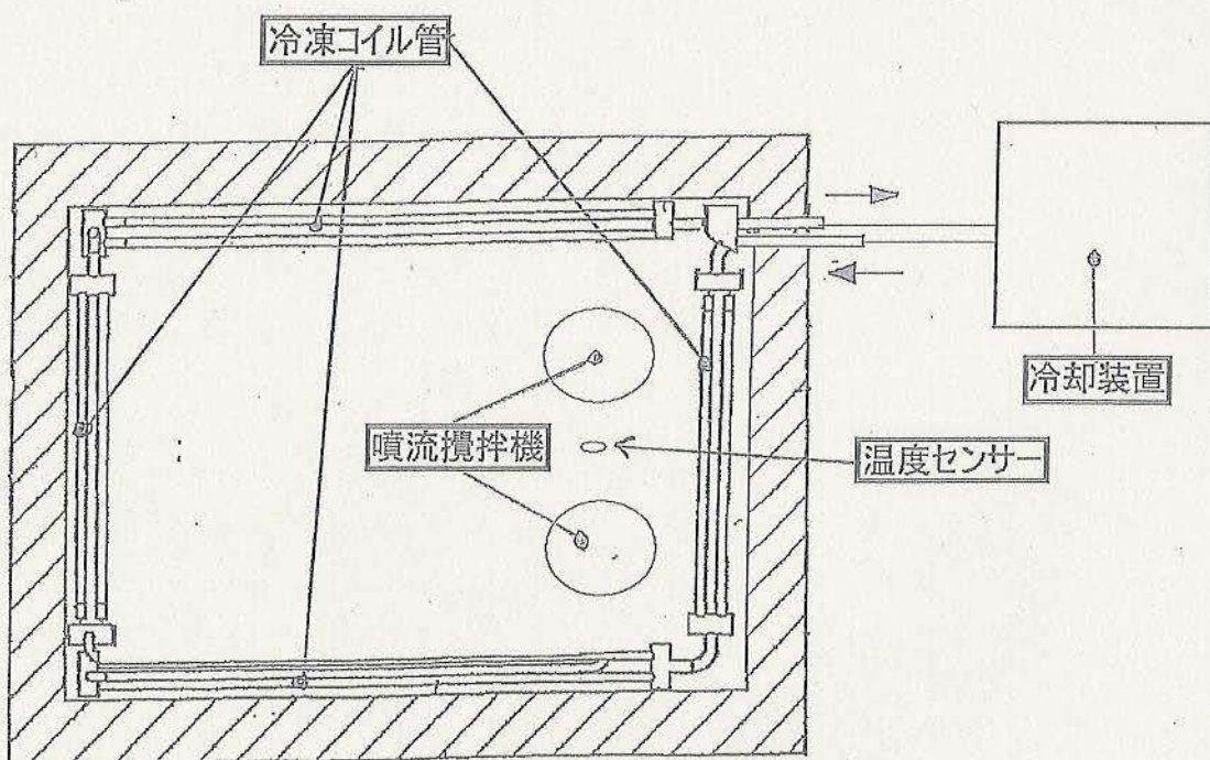
図面4 冷凍コイル管を示すための不凍液槽の平面断面図
