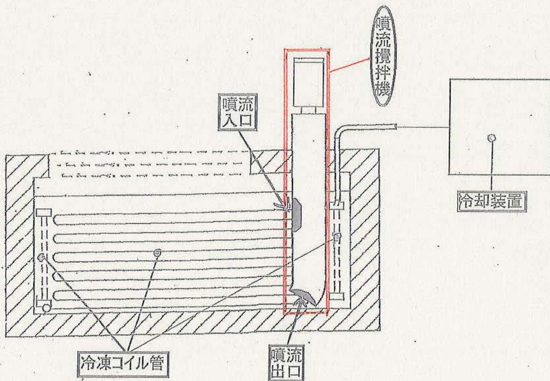
図面3 噴流攪拌機及び冷凍コイル管を示すための不凍液槽の正面断面図
