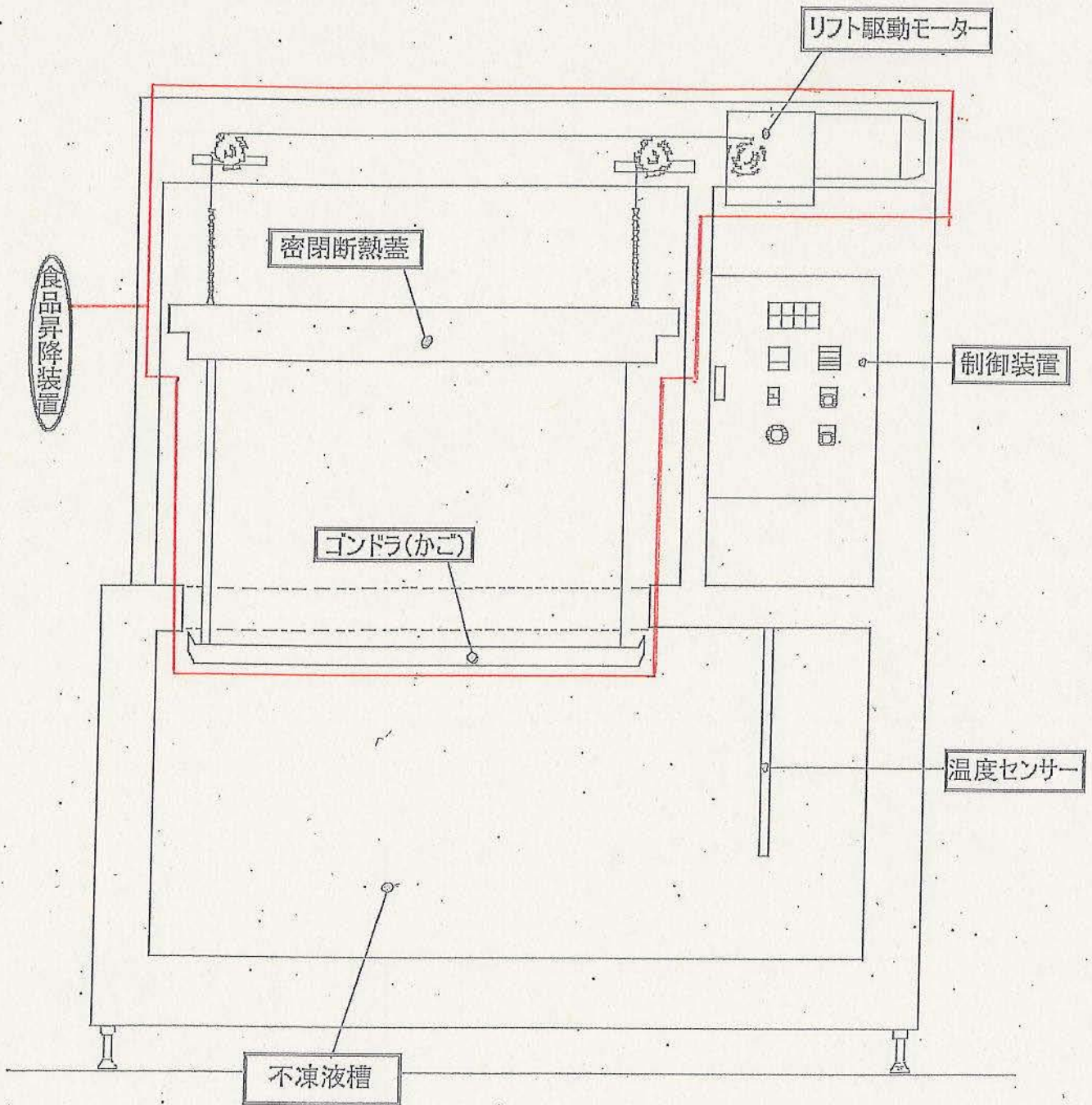
図面1 噴流攪拌機冷凍コイル管を除いた被告製品の正面図
