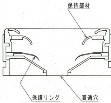
トレイ断面図
