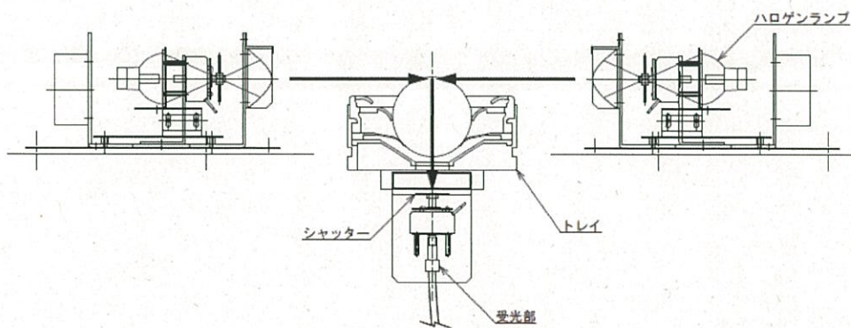
進行方向から見た側面拡大図
