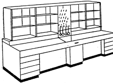
中央実験台 GF-Ⅲ型
