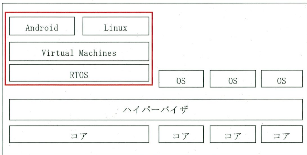
【図1：原告製品「MOS-S」「SecureOS」の構造】
