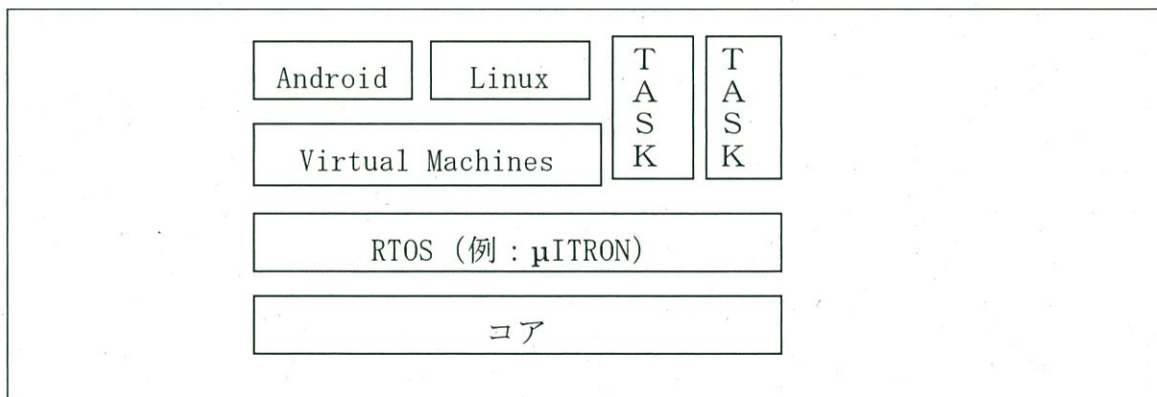
【図2：被告製品「EM-VRT」の構造】
