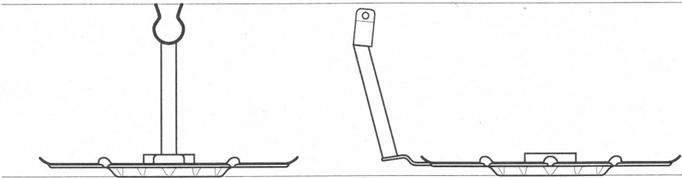
背面図
