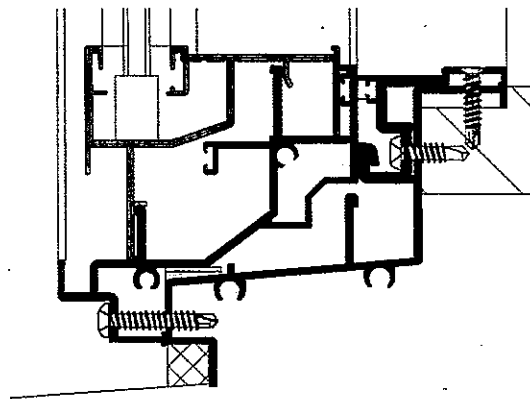
[下枠部分 X-X' 断面図]
