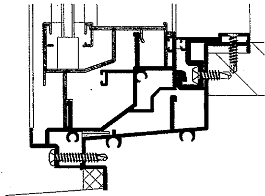
[下枠部分 Y-Y' 断面図]
