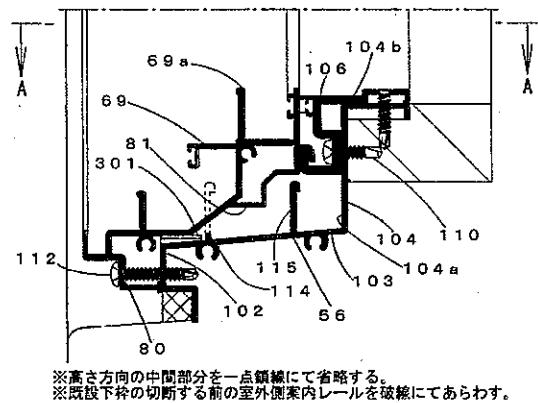
[下枠部分 X-X' 断面図]
