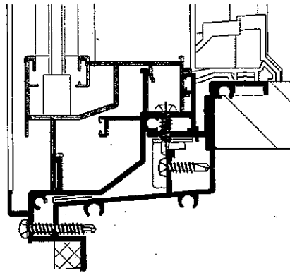
[下枠部分 X-X' 断面図]
