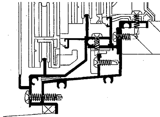
[下枠部分 X-X' 断面図]
