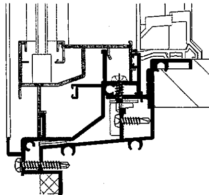
[下枠部分 Y-Y' 断面図]
