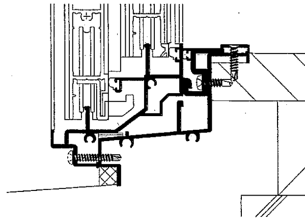
[下枠部分 X-X' 断面図]
