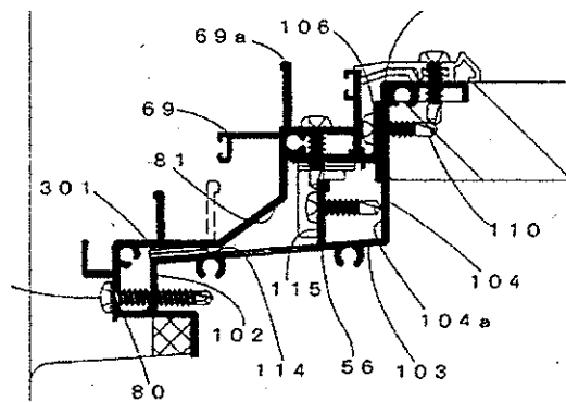
[下枠部分 X-X' 断面図]
