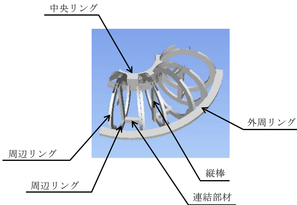
LL 型 部分詳細図
