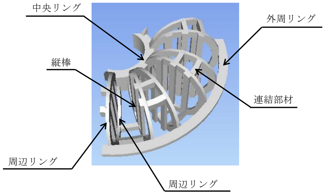
L-II型 部分詳細図
