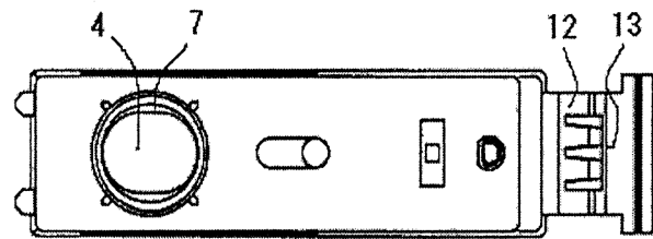
底面图 (第2图)
