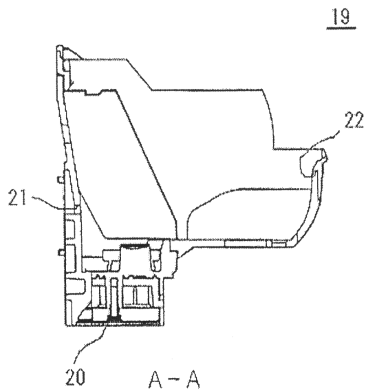
A-A線断面図 (参考図2)
