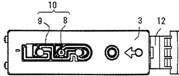
上面图 (第3图)
