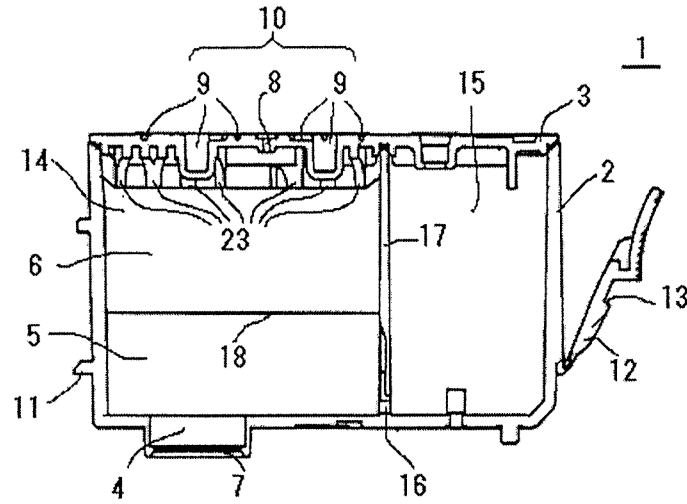
平面图 (第1图)
