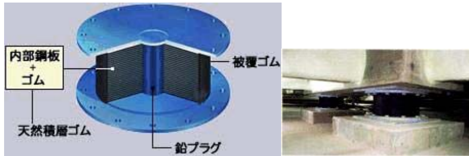
免震基礎
