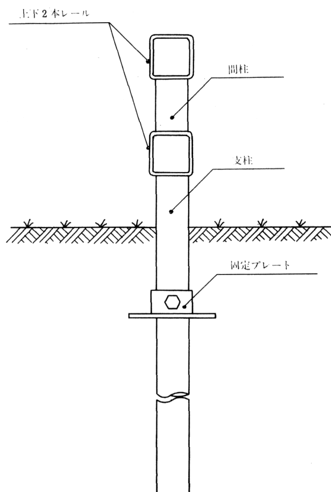
改良型、上下2本式レール設置図
