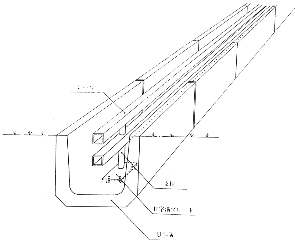
第7図 U字溝内の敷設方式説明図
