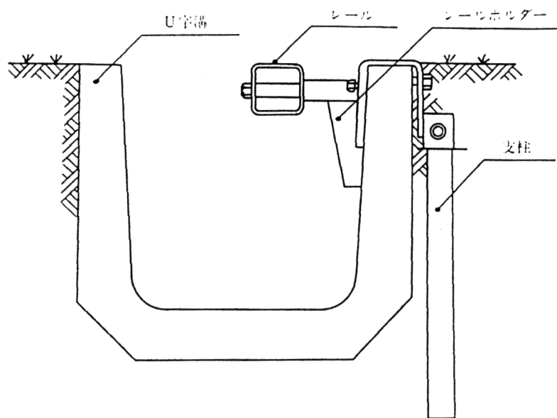
U字溝へ取付 モノレール工業種方式
