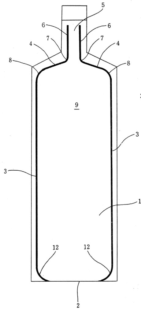
容袋のみの正面図
