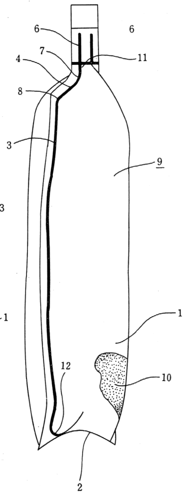
斜視図
