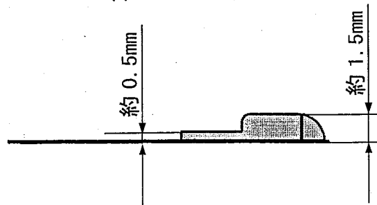
左側面拡大図
