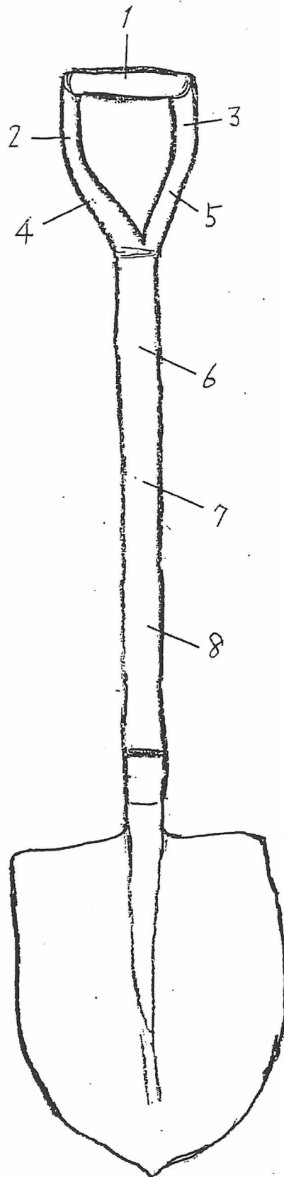
別紙 図面3 (本件スコップの略図)
