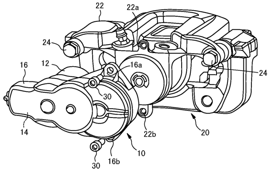
<図 1 : 被告製品の外觀図>
