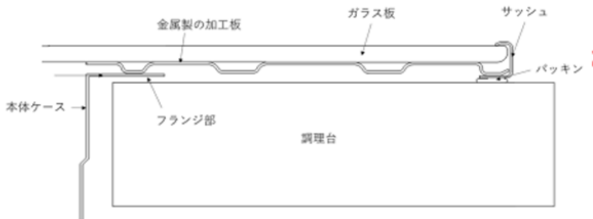
図5 BB断面図
