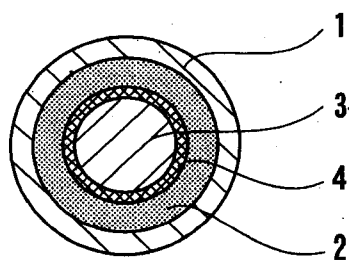
A-A断面図
