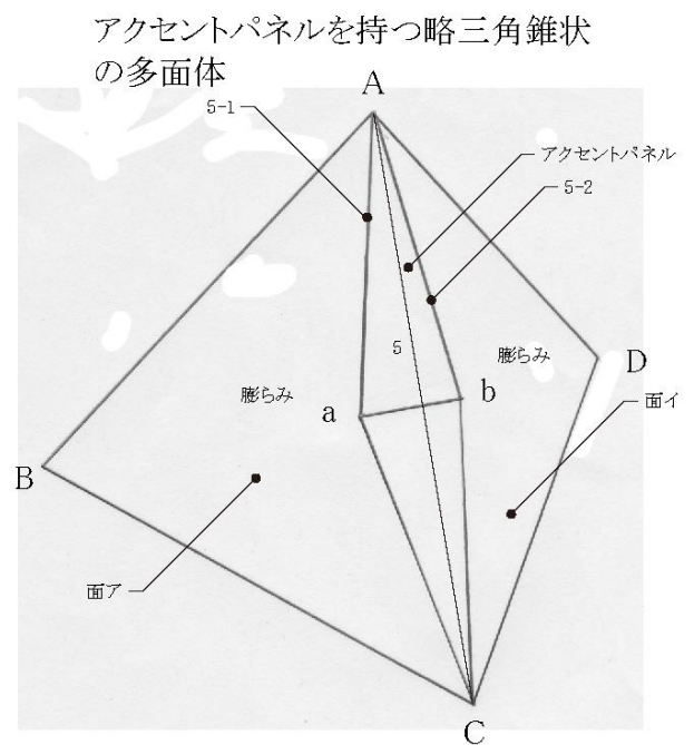
斜視図
