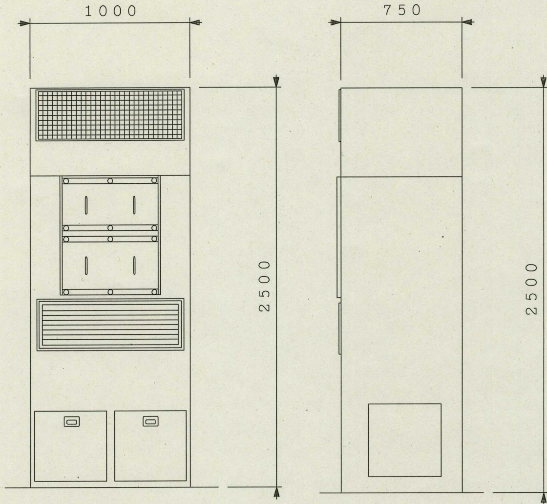
正面図
