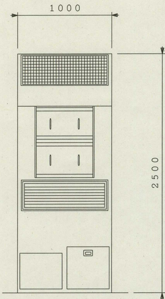
正面図
