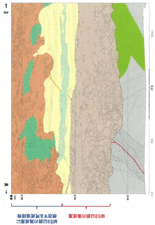
図表 3-2 F-1 断層付近拡大スケッチ
