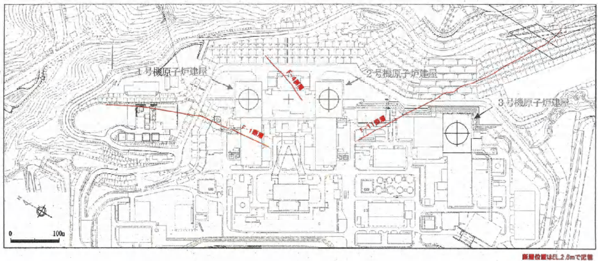
図表 1 - 2 F - 1 断層・F - 4 断層・F - 1 1 断層 平面位置図
