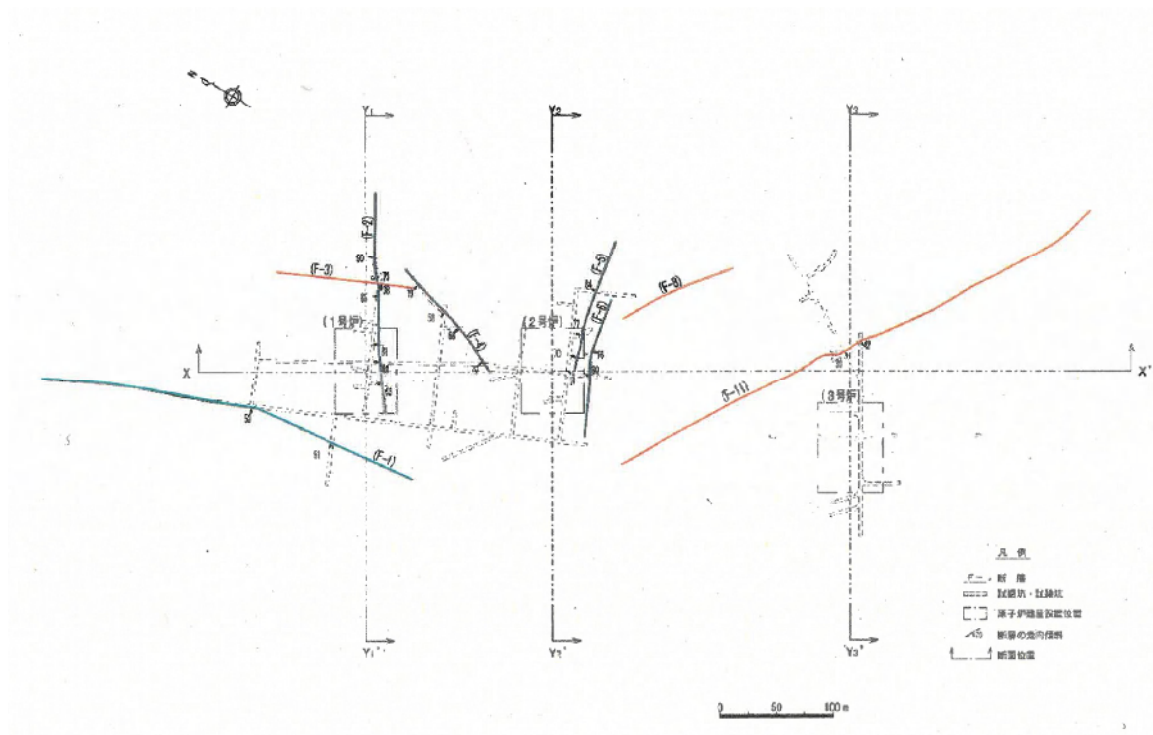
図表 1 - 1 断層平面位置図（断層位置は標高 2.8m で記載）
