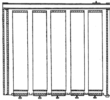
A-A線断面図
