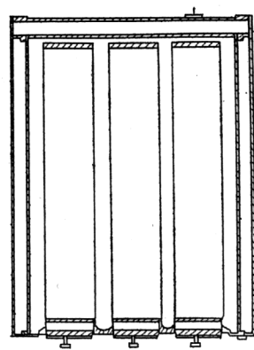
A-A線断面図
