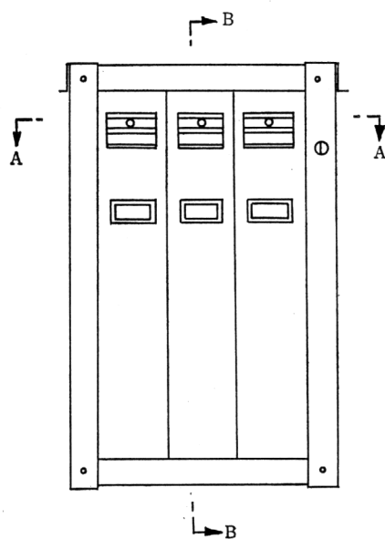
正 面 图
