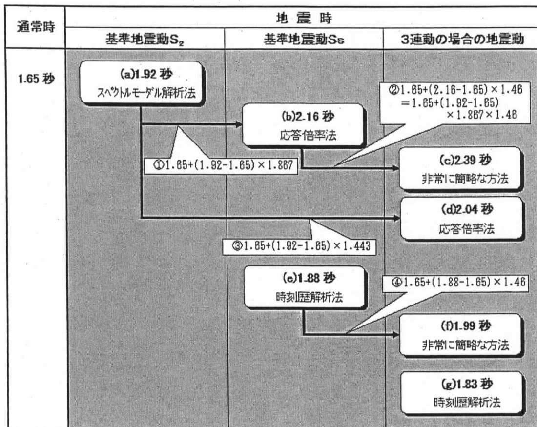
【図表 1 地震時の制御棒挿入時間】
