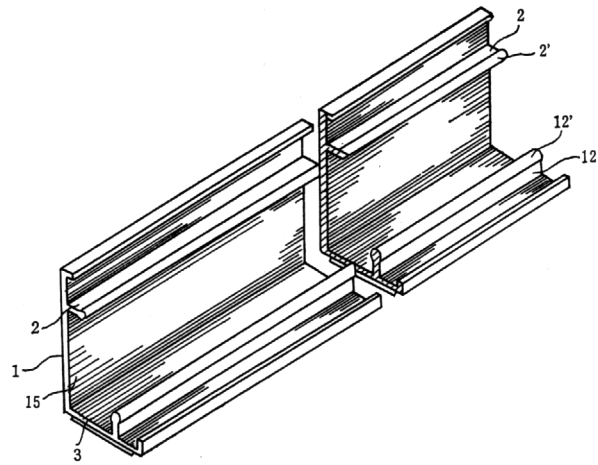
斜 視 図 (一部切欠)
