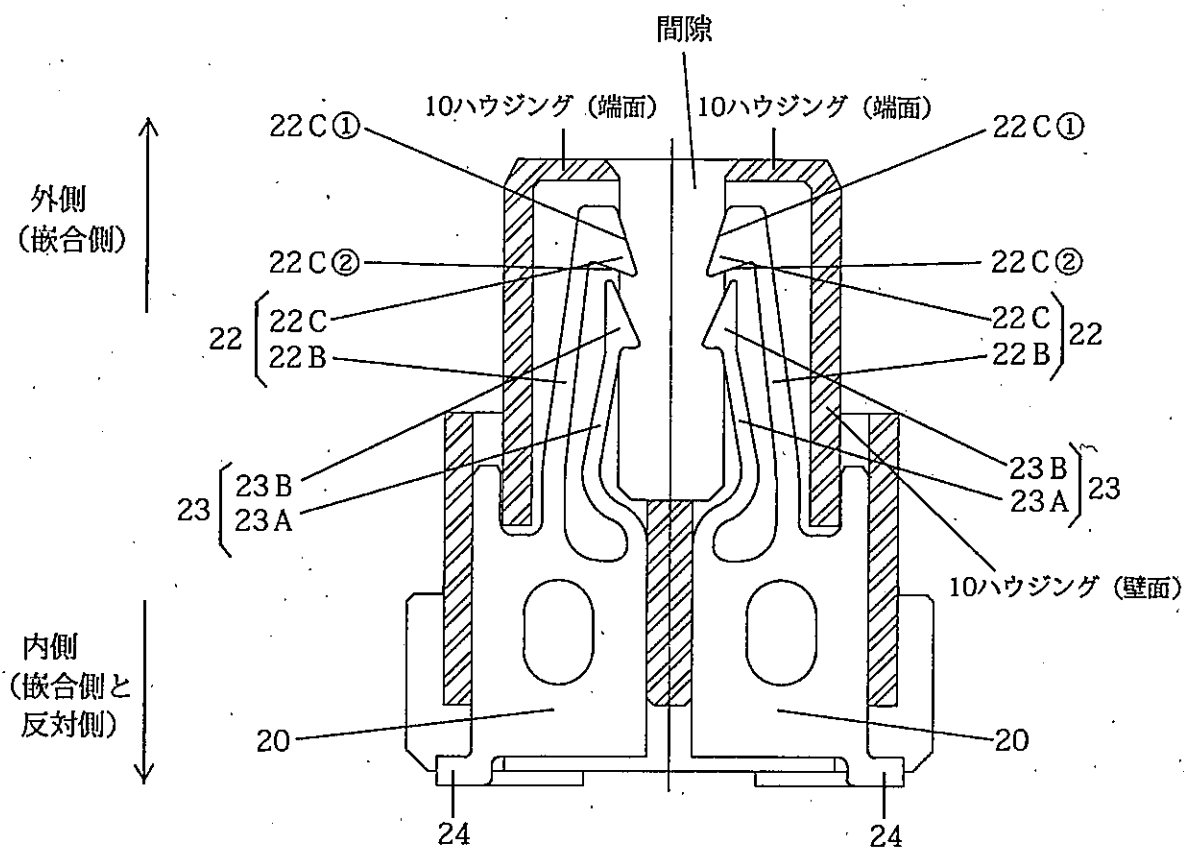
図 1 - 2 図 1 - 1 の A - A 断面図 (プラグ 3 0 と嵌合していない時)
