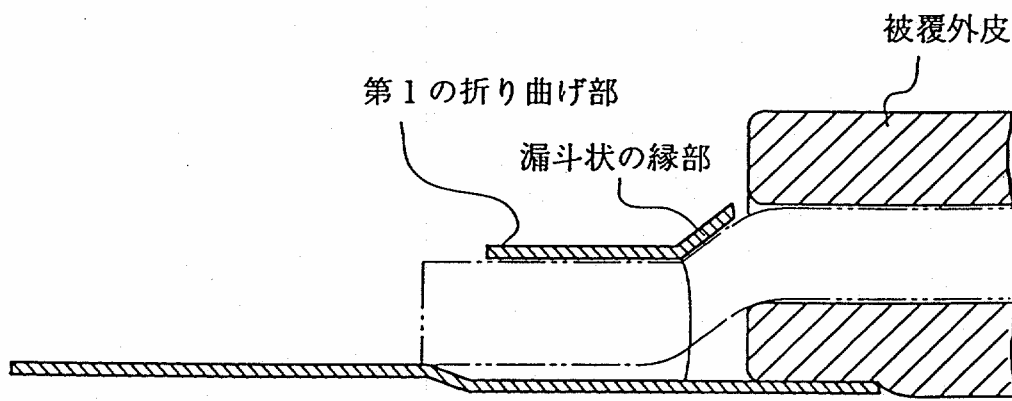
【図4】A—A断面図
