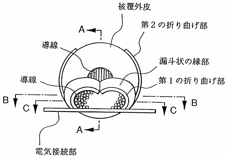
【図2】正面図
