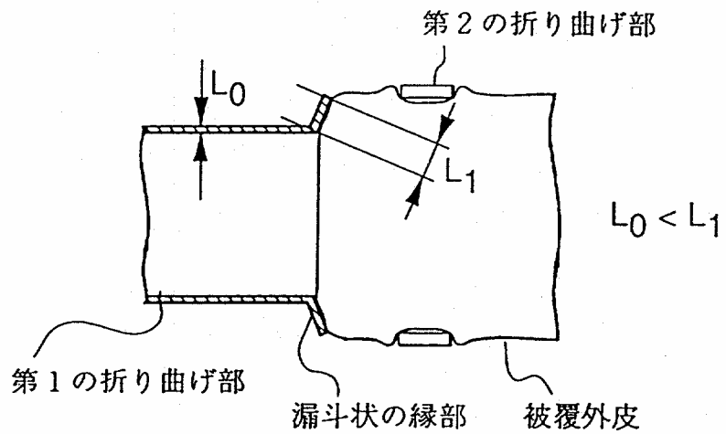
【図6】 C—C断面図
