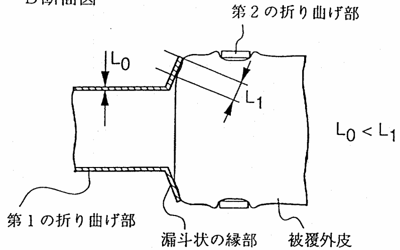
【図5】 B—B断面図
