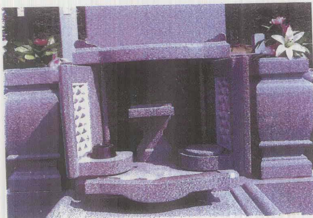
(2) 収納箱前面を開口した状態の正面図
