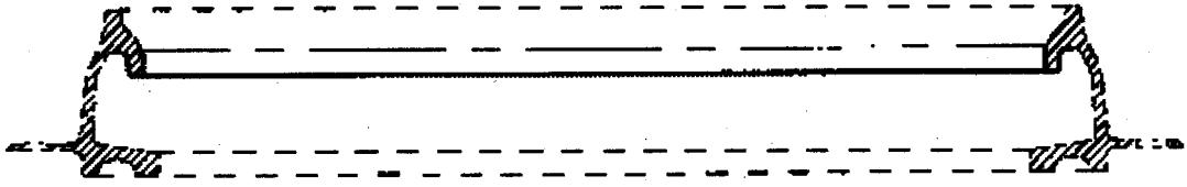
【D-D扩大端面图】
