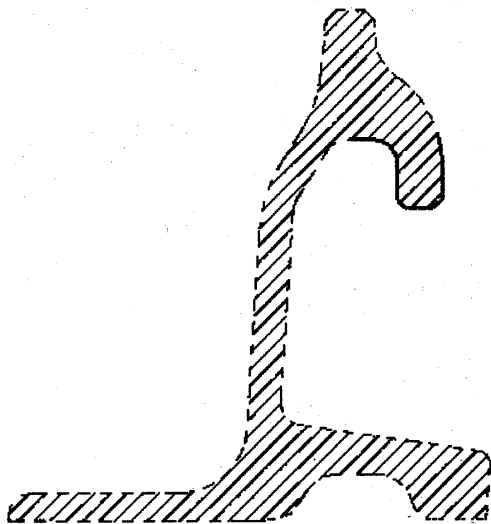
【E—E扩大端面图】
