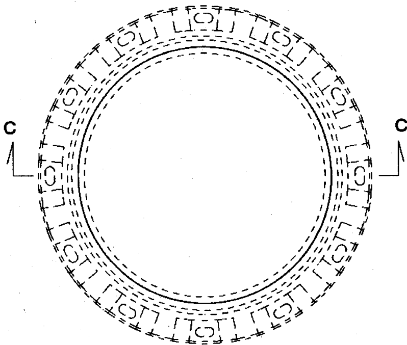
【A-A断面图】
