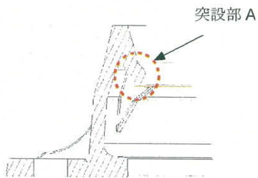
(10) E-E 拡大図
