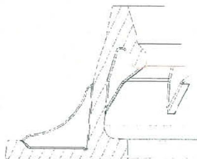
(10) E-E 拡大図
