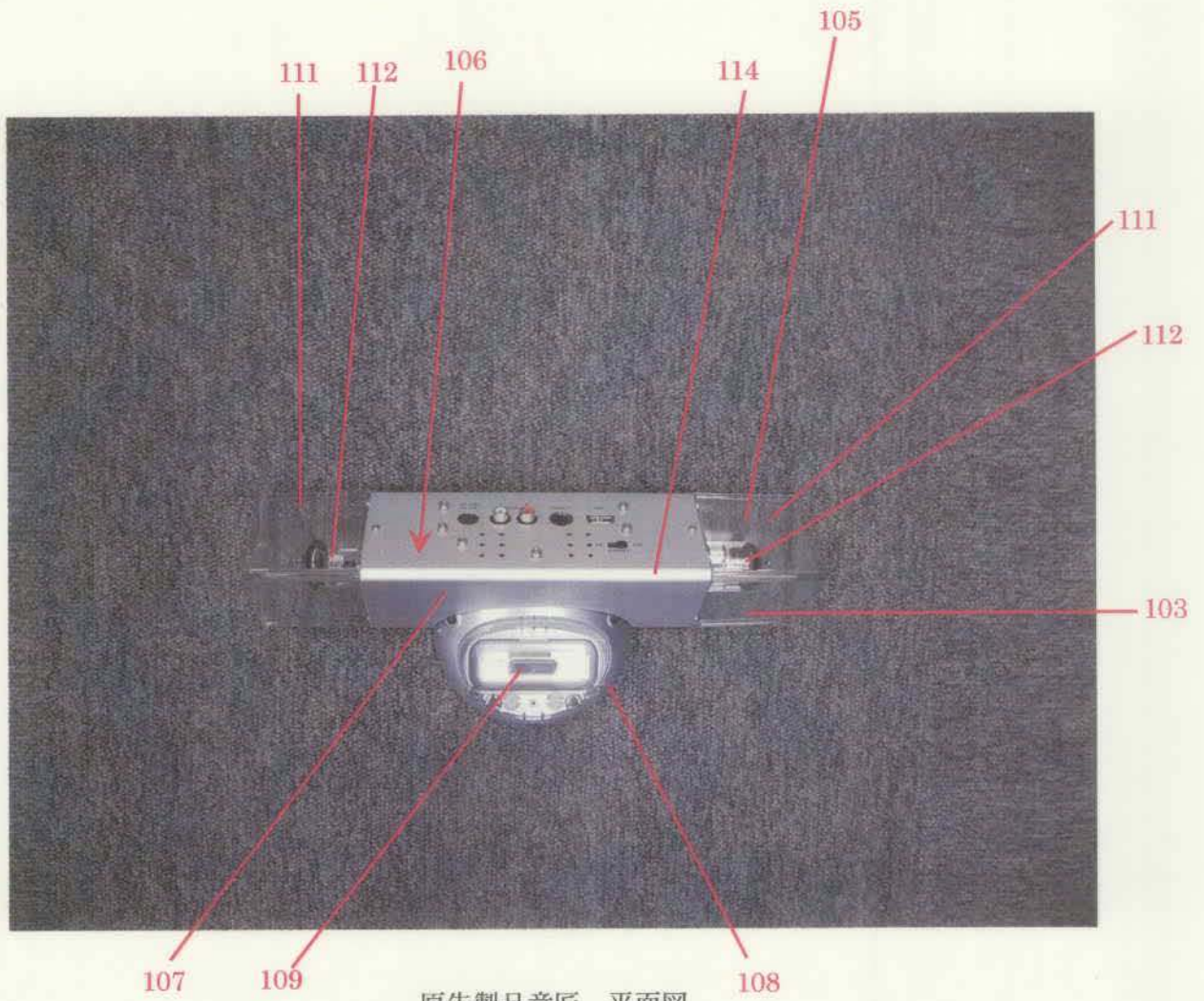
原告製品意匠 平面図
