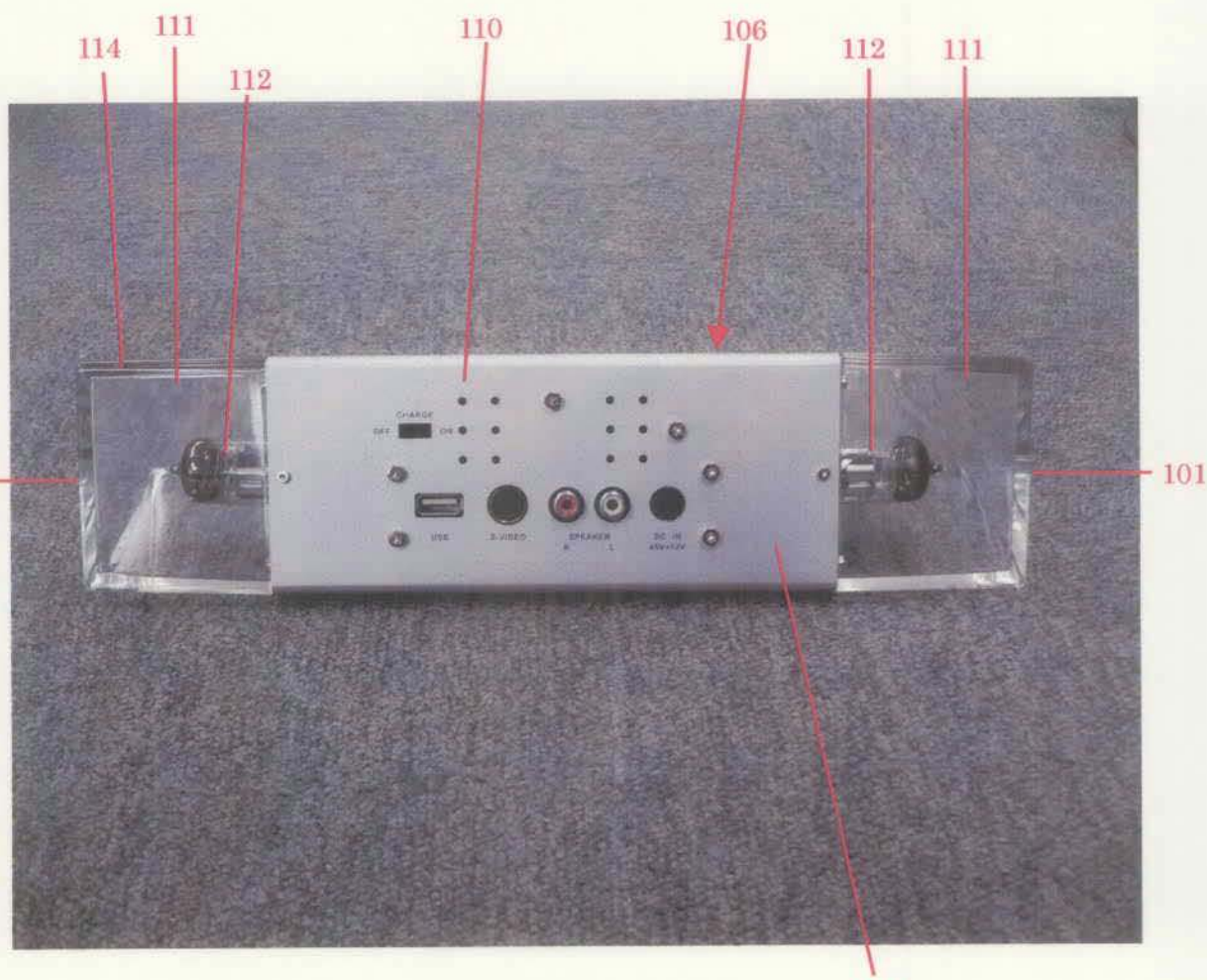
原告製品意匠 背面図
