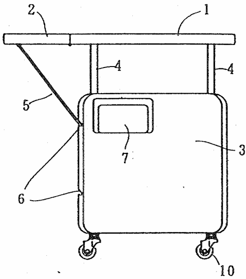
正面図
