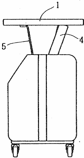
右側面図
