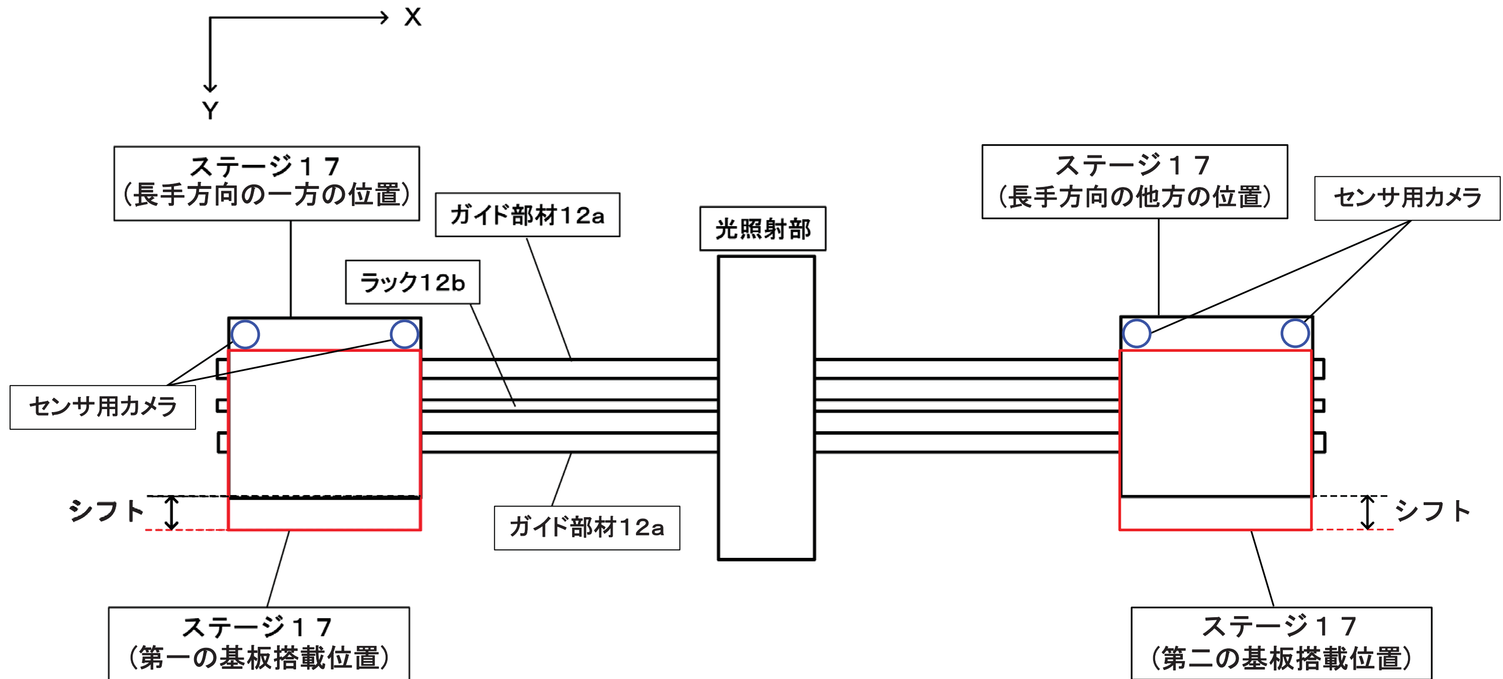
図 1 (平面図)
