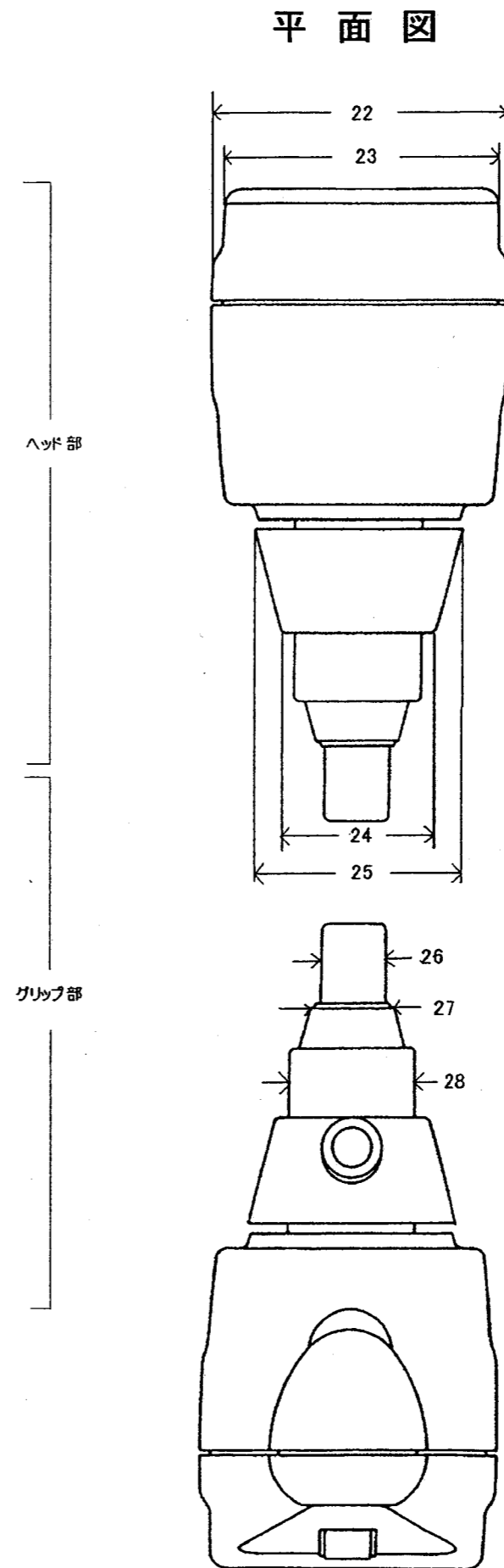
底面図
