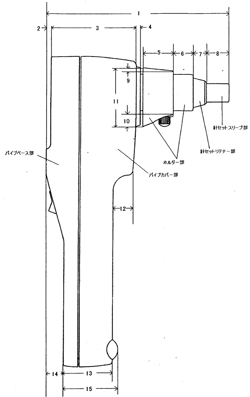
側面図
