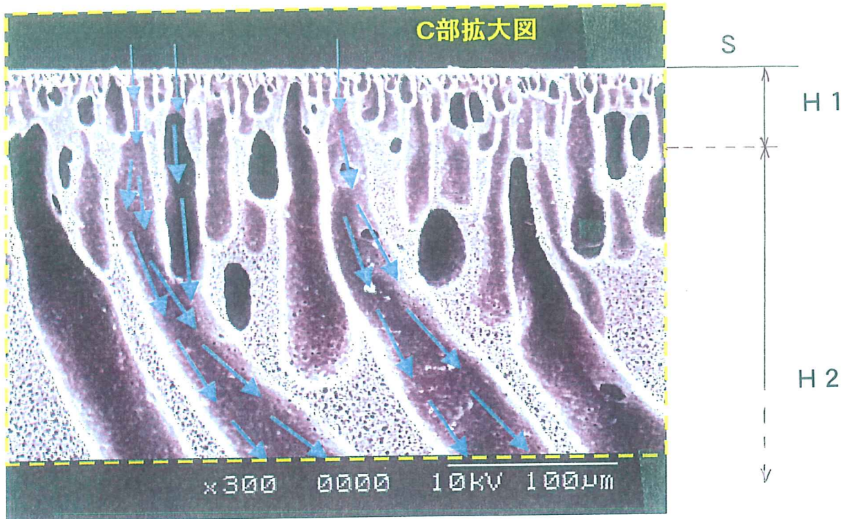
図 1のC部拡大図 300倍
