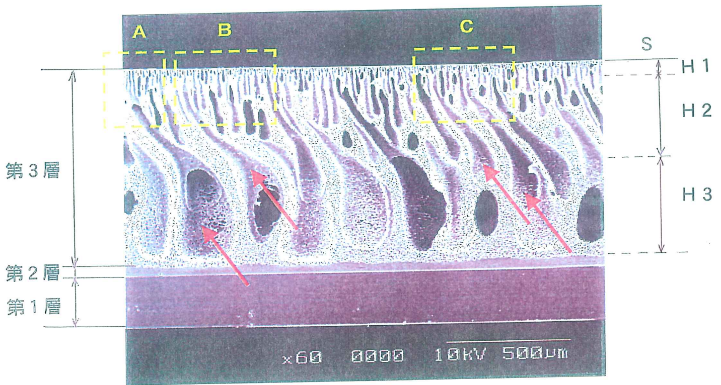
NP025断面 60倍SEM
