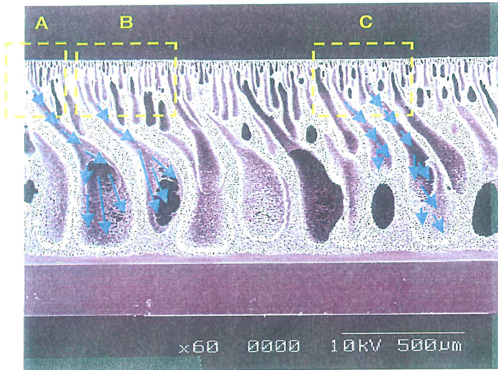
NP025断面 60倍 (图中→ は、発泡形成時の成長方向)
