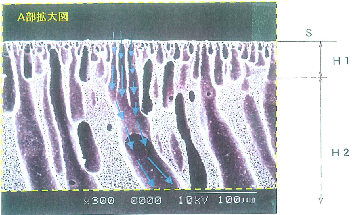
図 1のA部拡大図 300倍
