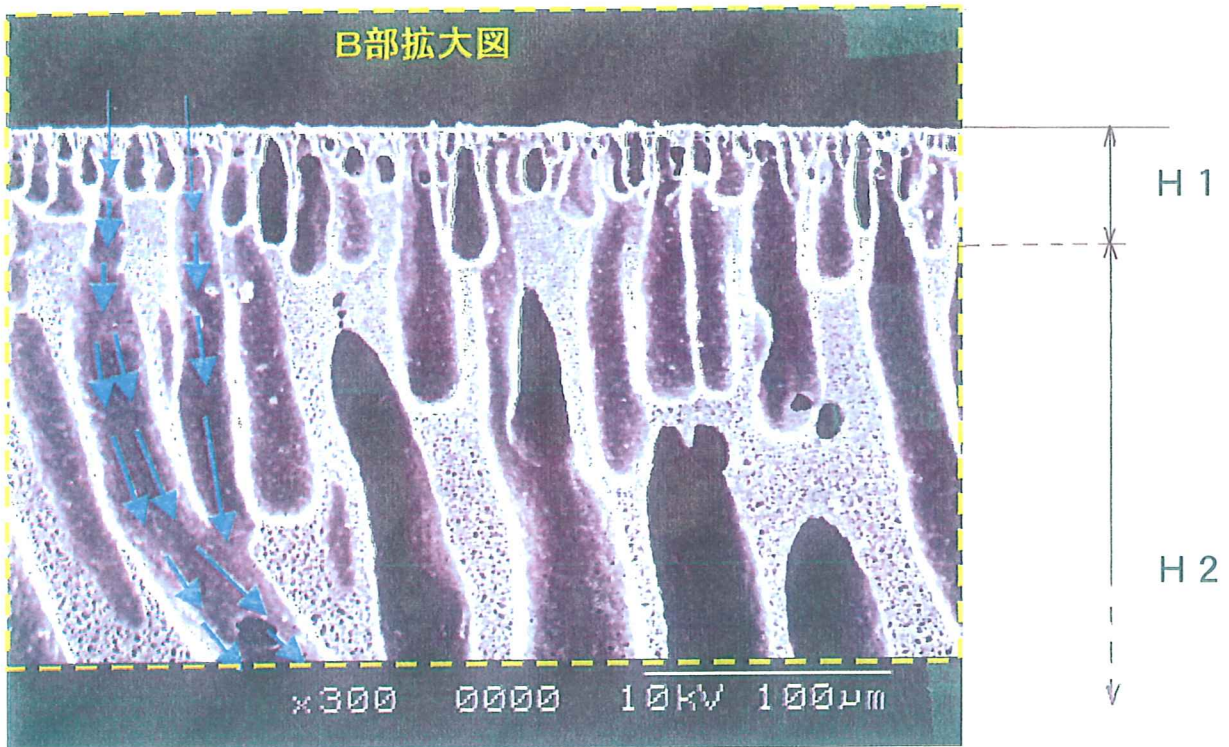
図 1のB部拡大図 300倍
