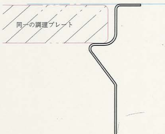
C：松岡製作所 3DMシンクのリブ
