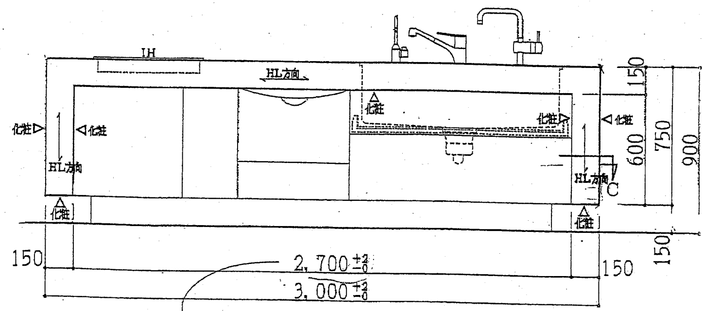
正面図 S=1/20
