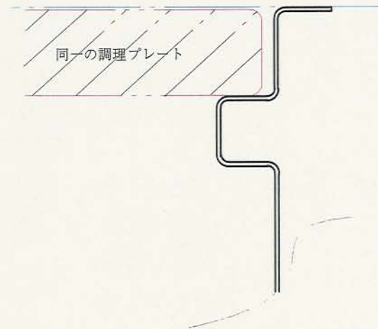
B：四角のリブ
