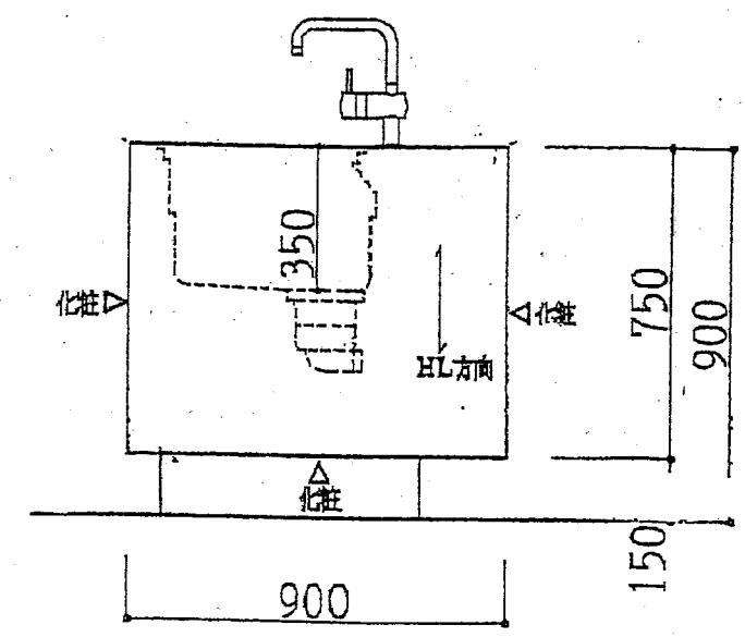
側面図 S=1/20
