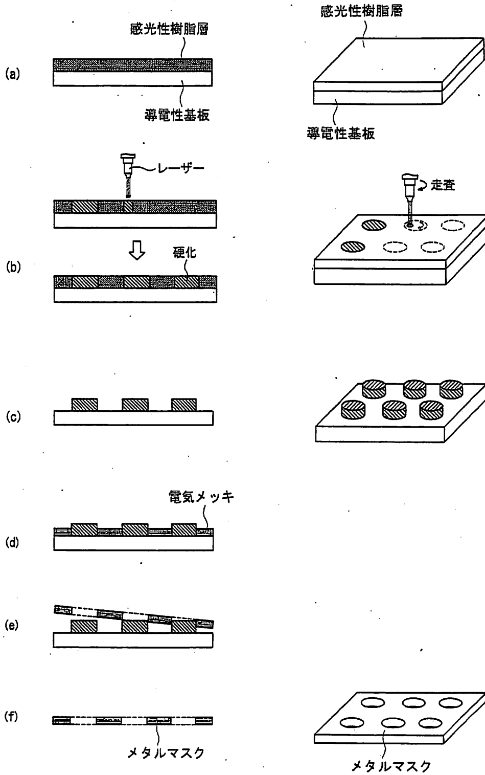
図1 本願発明によるメタルマスク製造法
