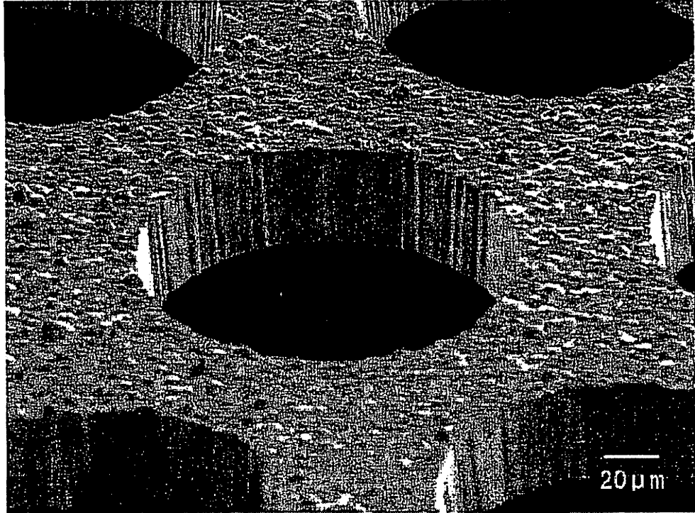
図2 従来技術により製造されたメタルマスク
