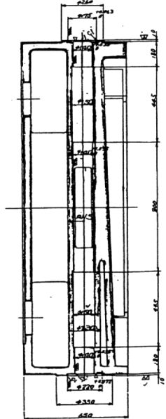
断面 D-D
