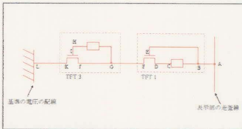
説明図2：写真14中のTFT1及びTFT3に着目した回路を抜き出した回路図
