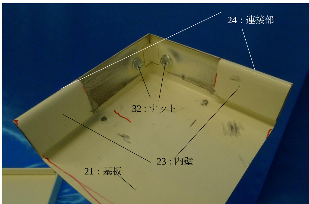
図9 CSスーパーワゴンの棚板のコーナー部付近を、内壁及び接続部を切り欠いて、側斜め上から見た図
