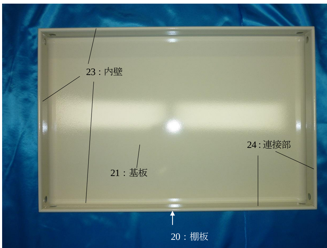
図4 CSスーパーワゴンの棚板を上から見た図
