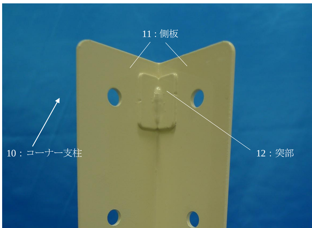
図2 CSスーパーワゴンの支柱を内側から見た図
