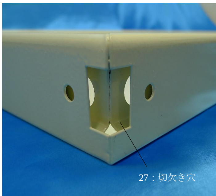
図6 CSスーパーワゴンの組立前の棚板のコーナー部分を外側から見た図
