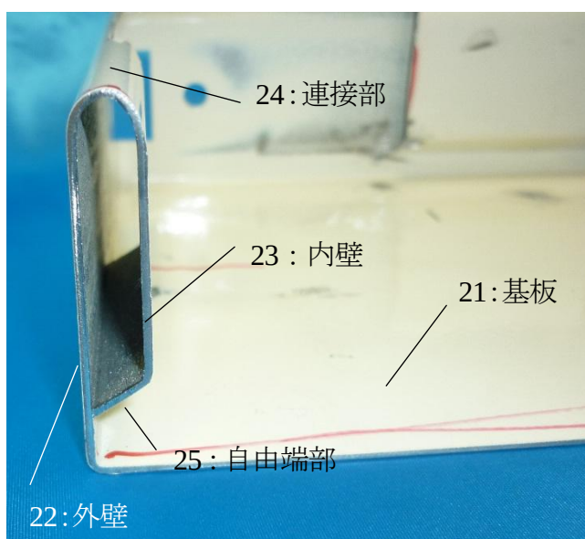
図5 CSスーパーワゴンの棚板の断面図
