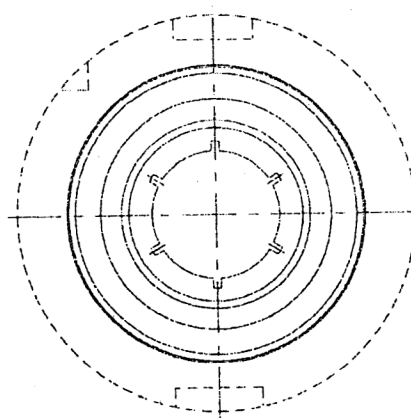
右側面図
