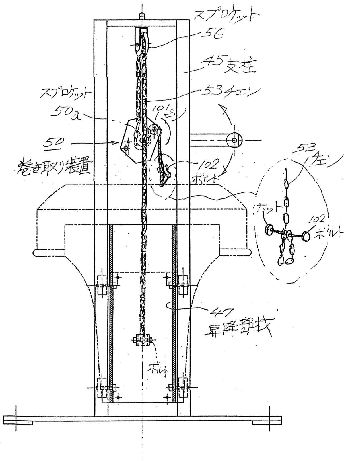
II-II 矢視図
