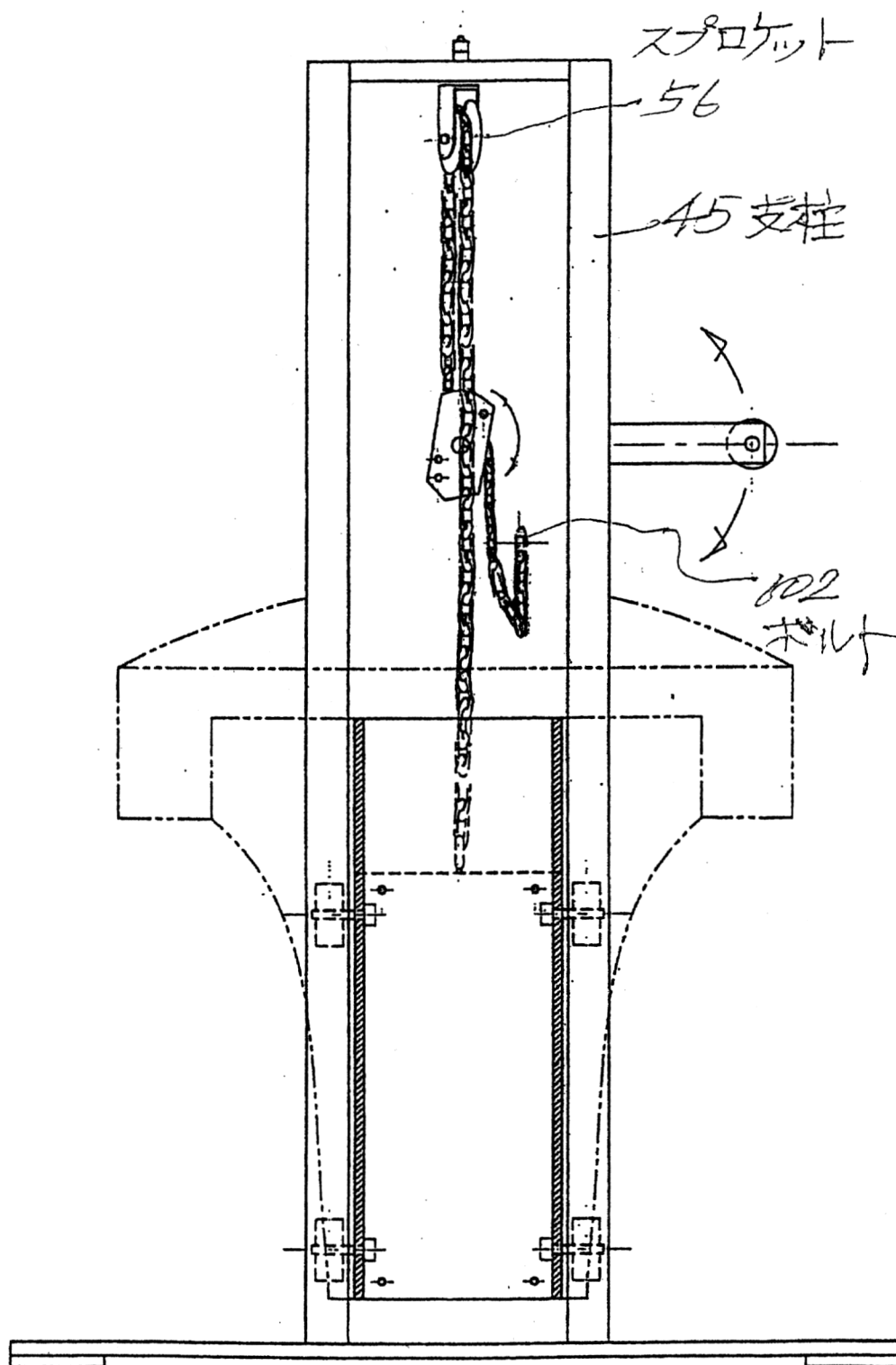
II-II 矢視図
