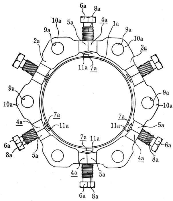
背面图
