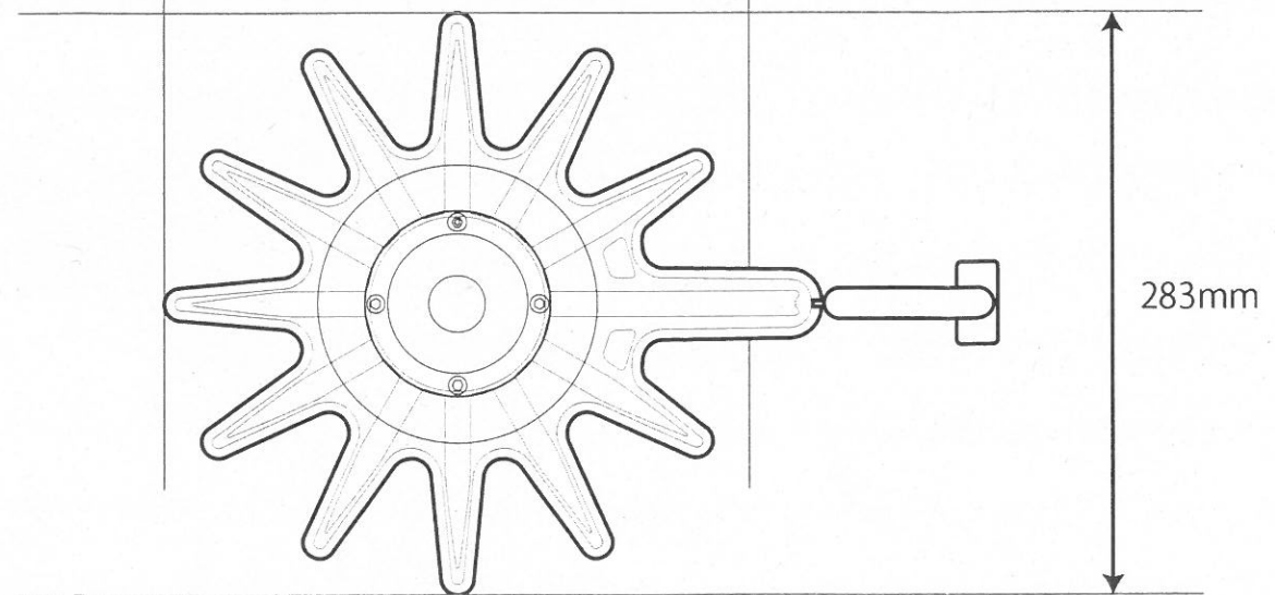
底面図
