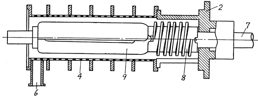
第4図 精白室横断平面図
