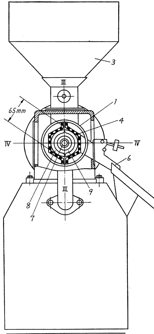
第2図 縦断正面図
