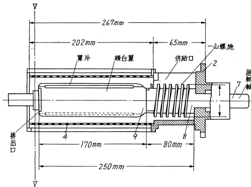
第3図 精白室縦断側面図
