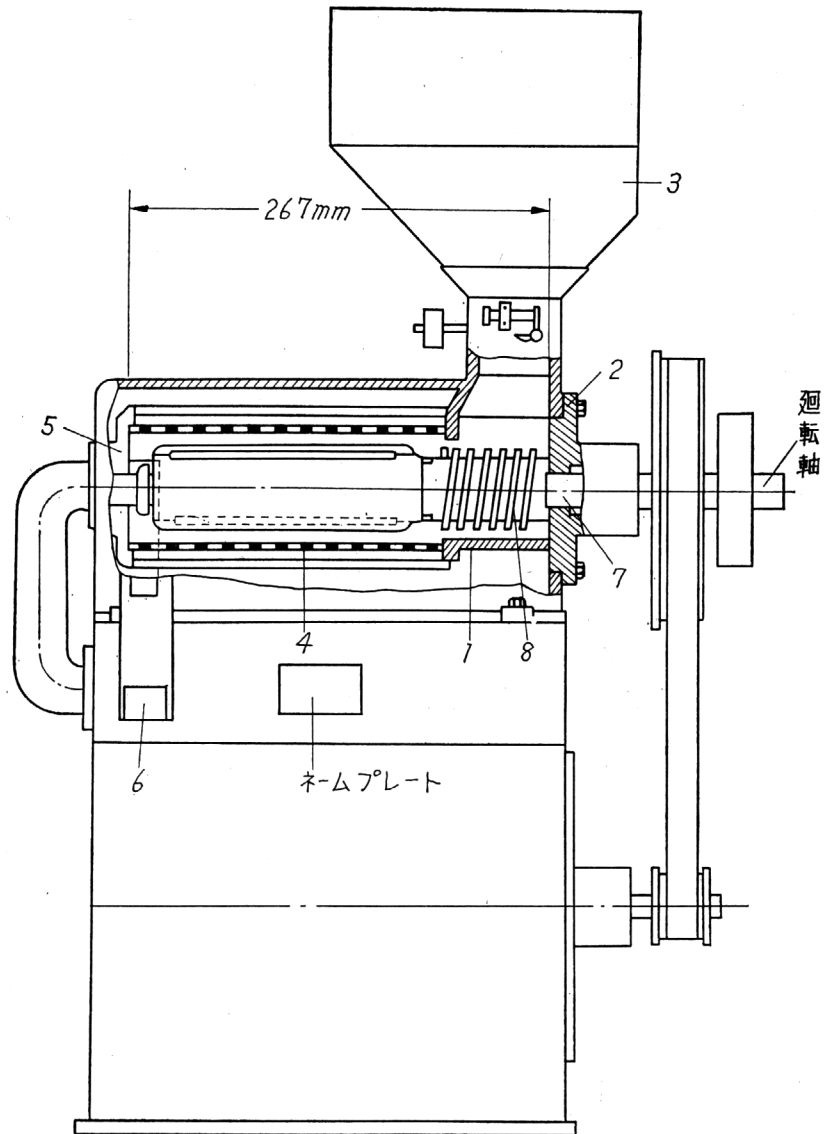
第1図 縦断側面図
