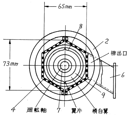
第5図 精白室縦断正面図
