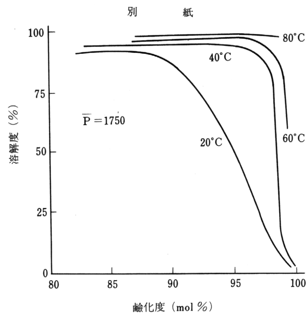
図2 鹼化度と溶解度
