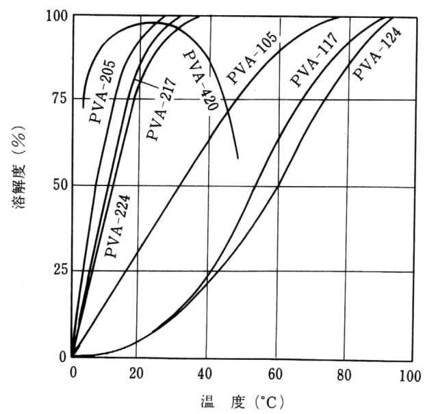
図3 温度と溶解度
