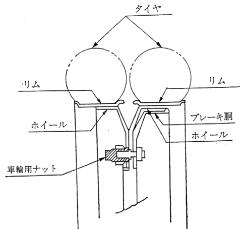
参考図
